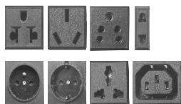
Optional sockets
